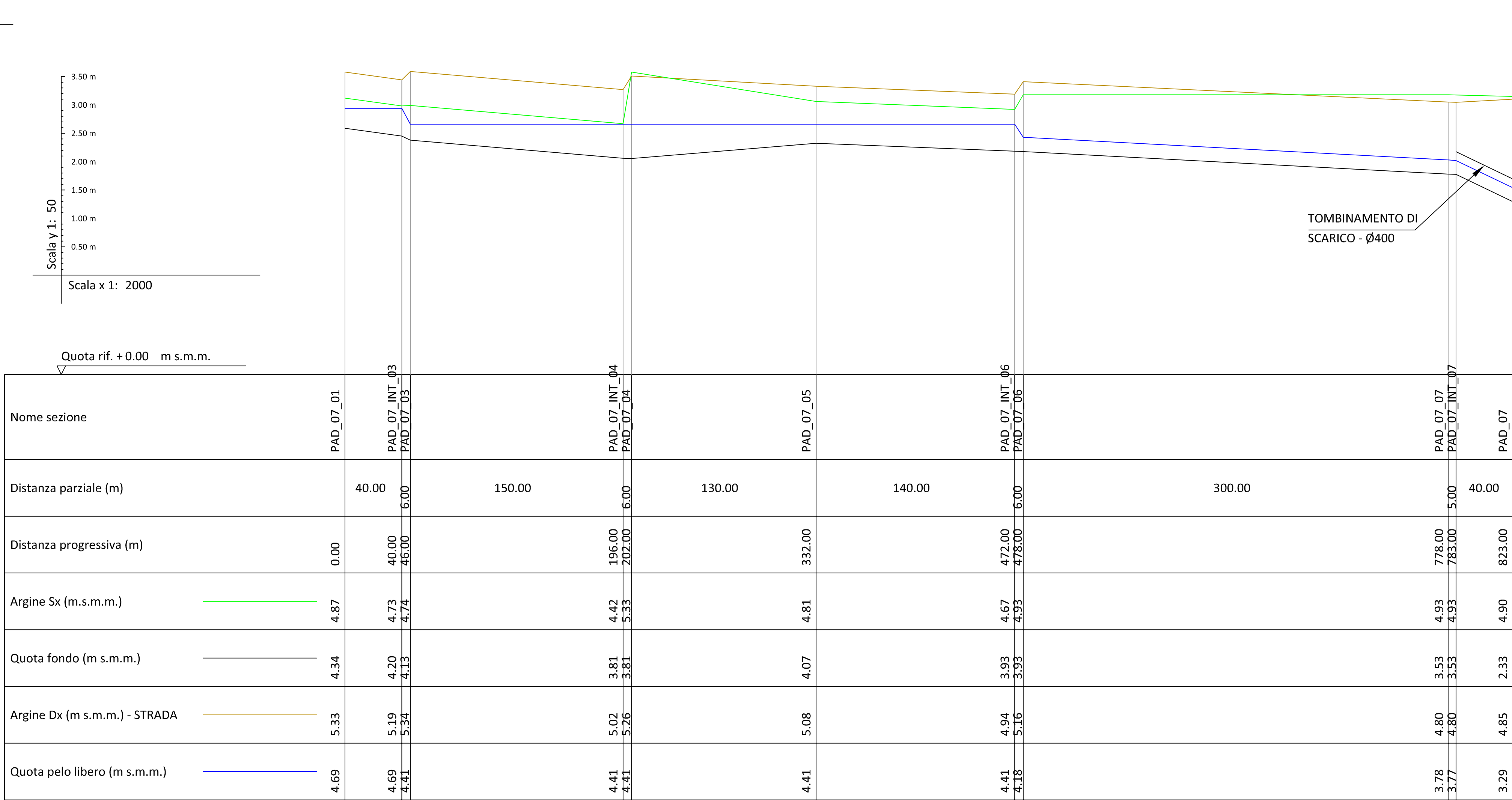
PROFILO LONGITUDINALE PAD_07_ii VIA GALLI TEMPO DI PIOGGIA 1 h Tr = 20 anni
