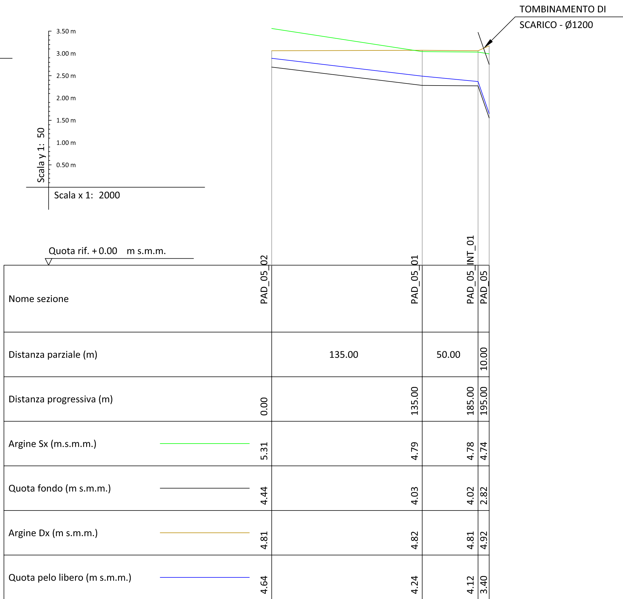
PROFILO LONGITUDINALE PAD_05_ii TEMPO DI PIOGGIA 1 h Tr = 20 anni
