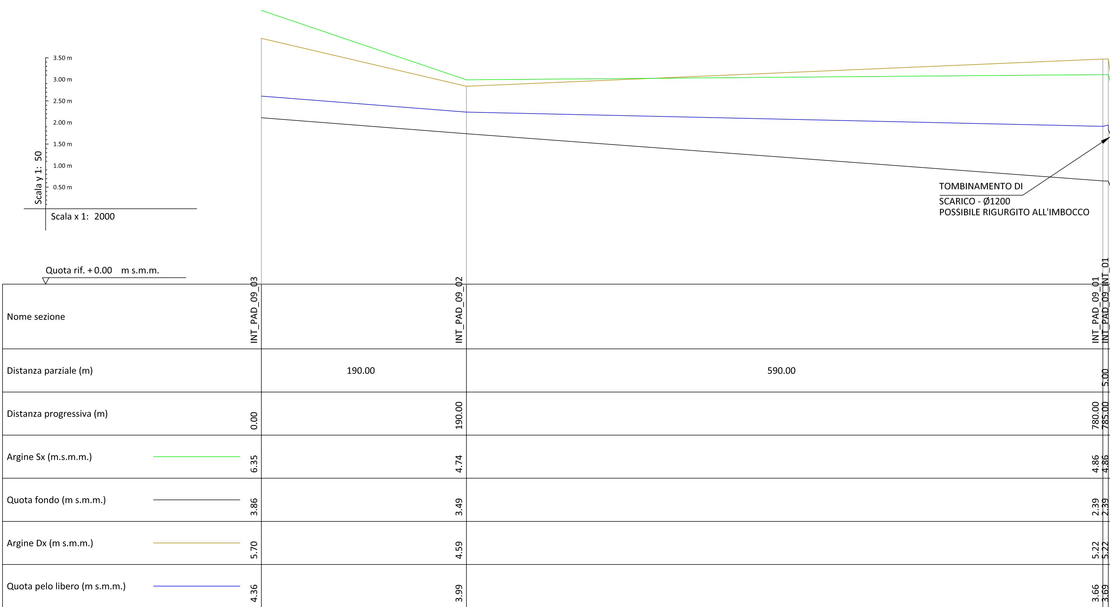
PROFILO LONGITUDINALE INT_PAD_09_ii TEMPO DI PIOGGIA 1 h Tr = 20 anni
