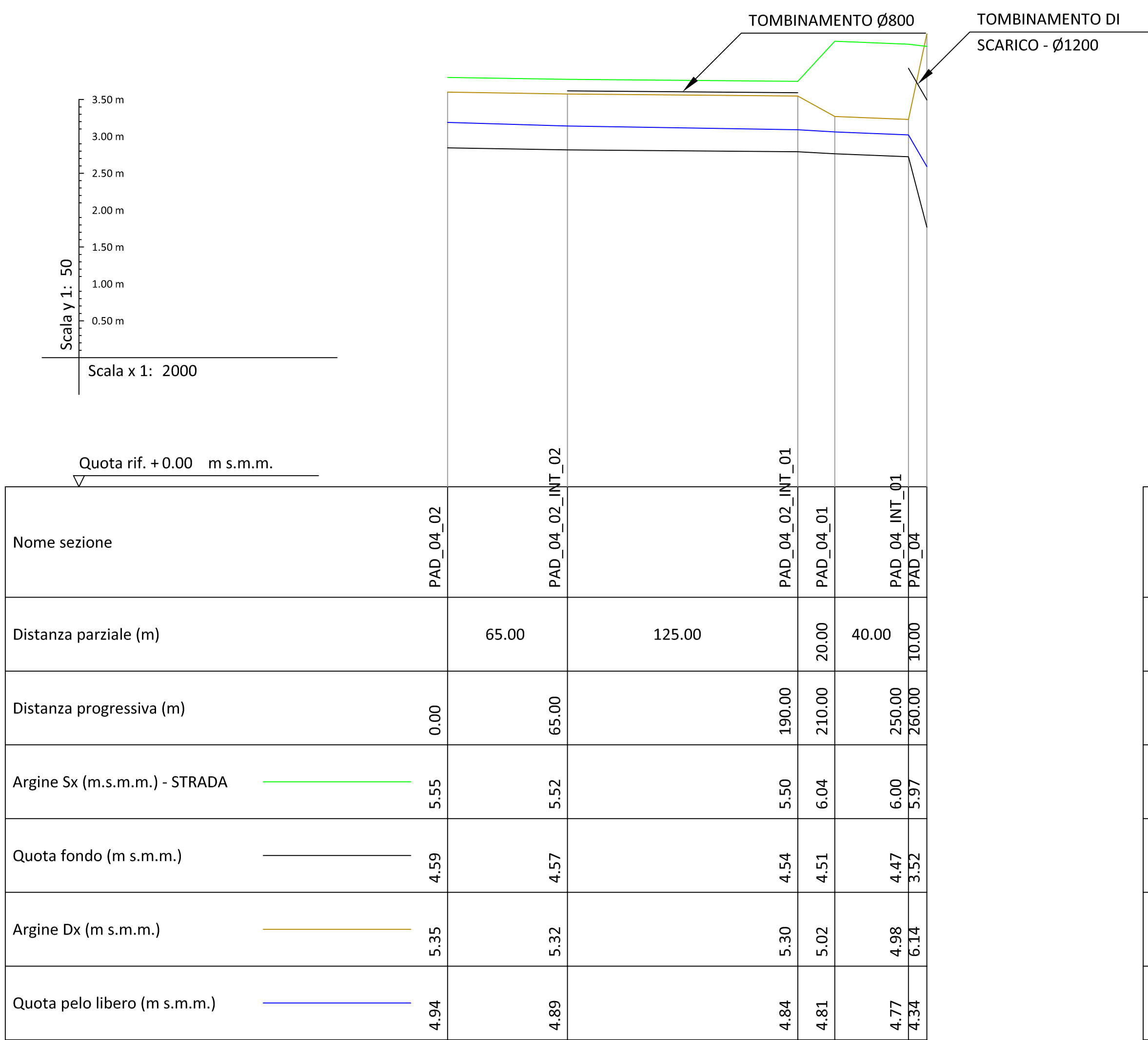
PROFILO LONGITUDINALE PAD_04_ii TEMPO DI PIOGGIA 1 h Tr = 20 anni
