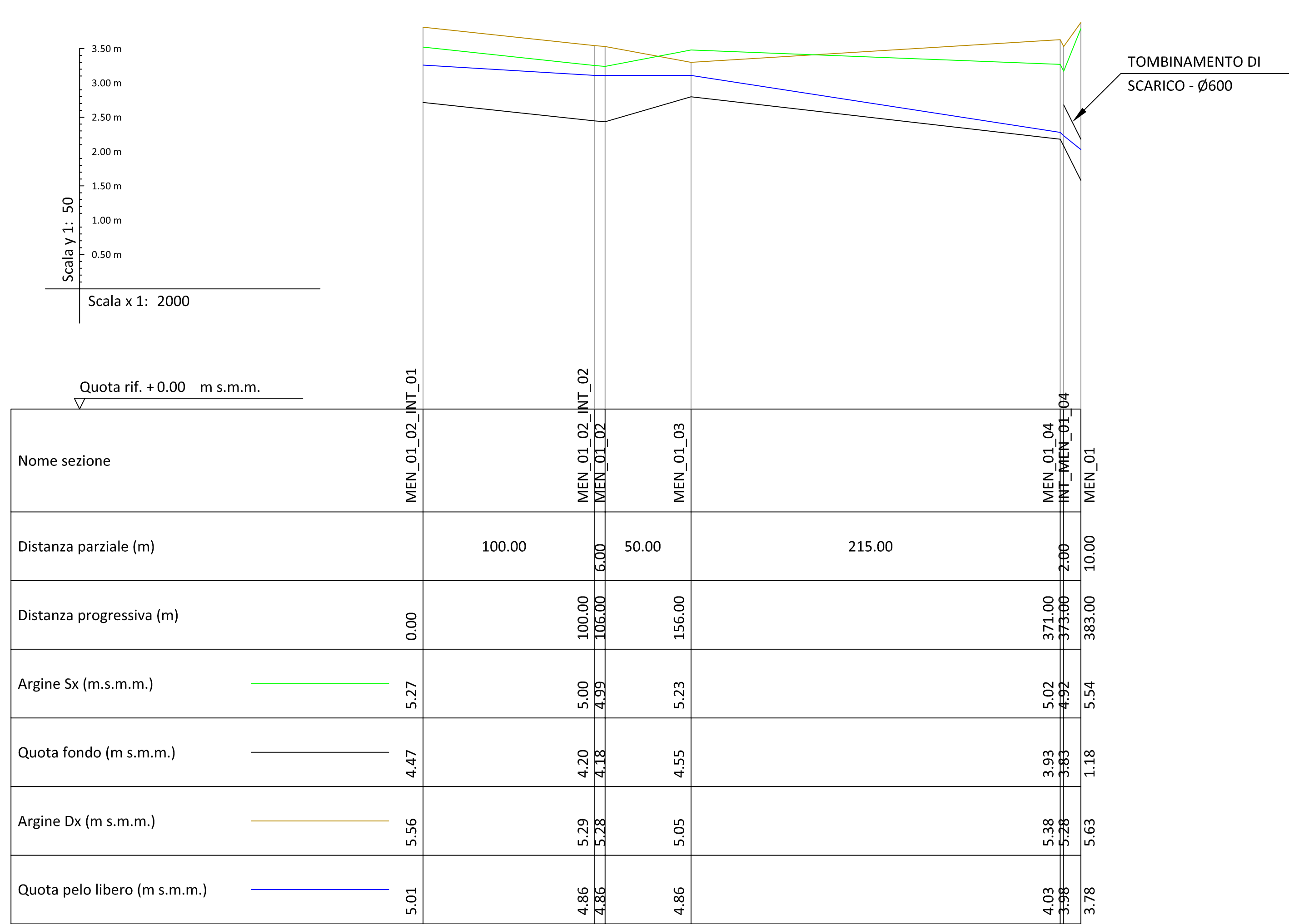
PROFILO LONGITUDINALE MEN_01_1 TEMPO DI PIOGGIA 1 h Tr = 20 anni
