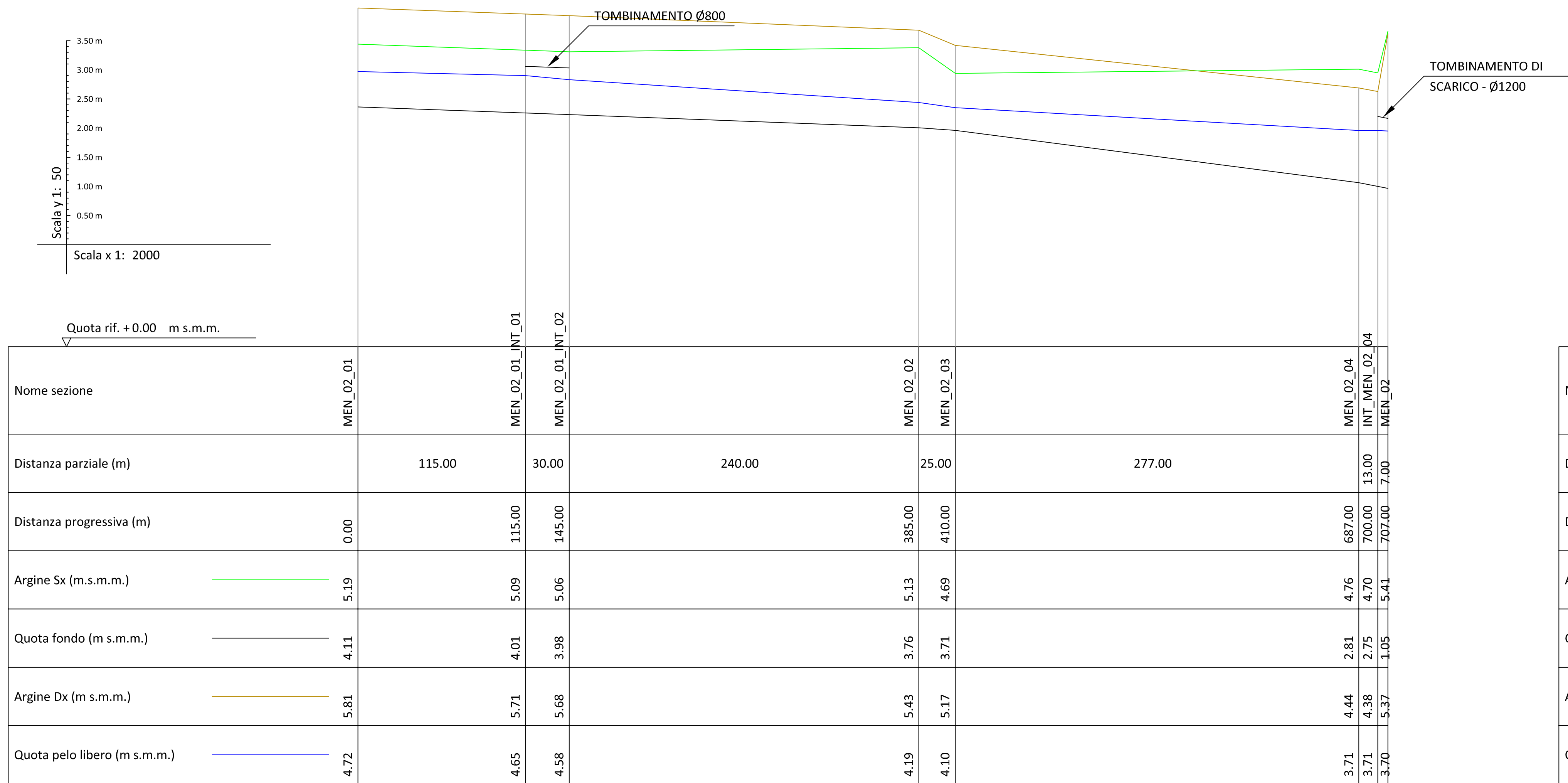
PROFILO LONGITUDINALE MEN_02_ii TEMPO DI PIOGGIA 1 h Tr = 20 anni
